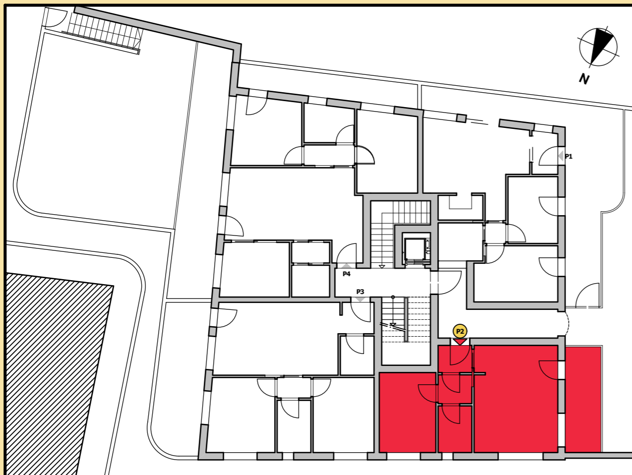
Lageplan Erdgeschoss
