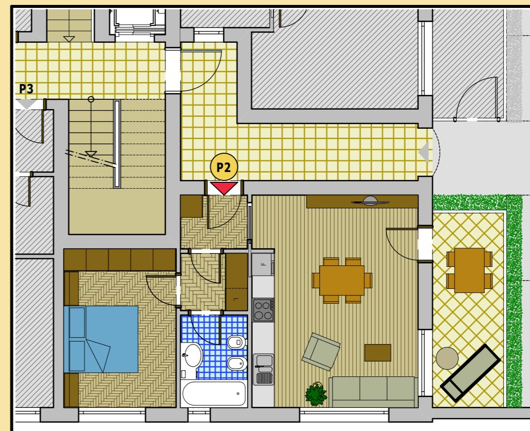
Erdgeschoss
