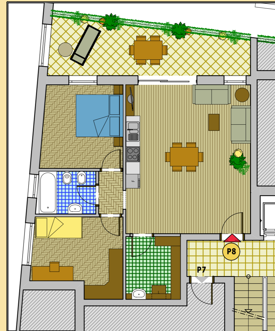
1. Obergeschoss
